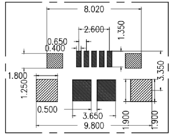
PCB参考图
